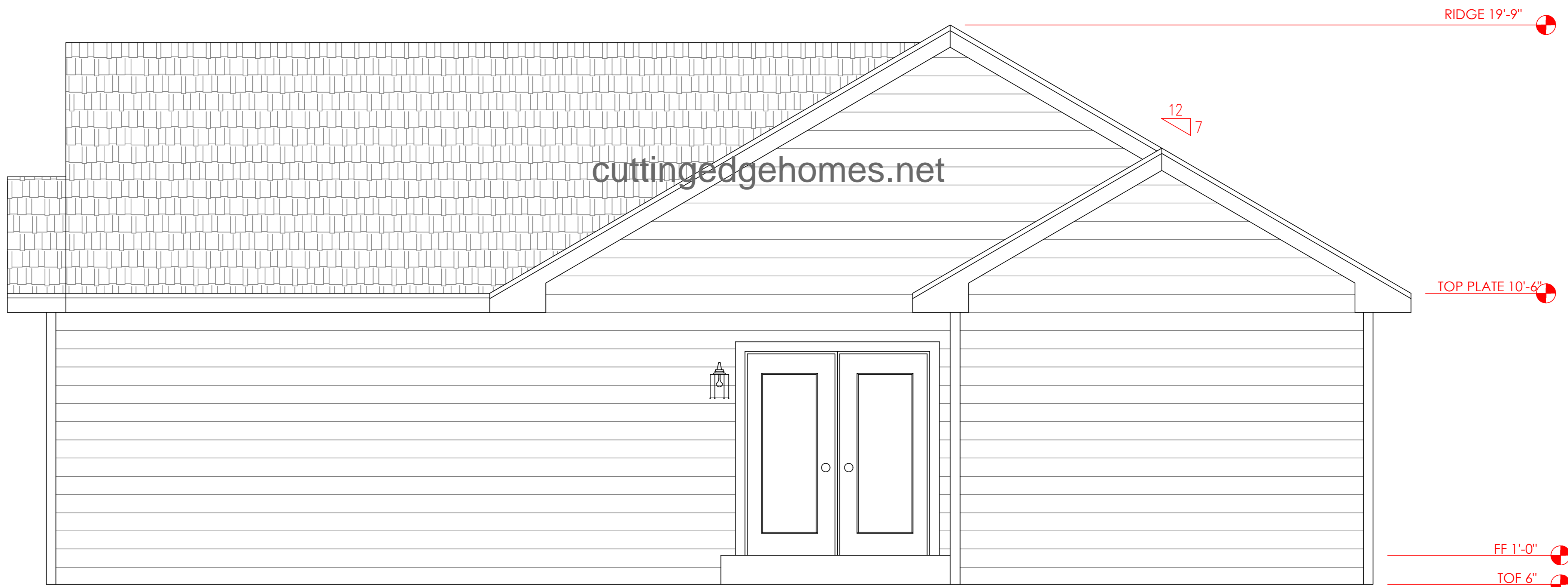
RIGHT ELEVATION
